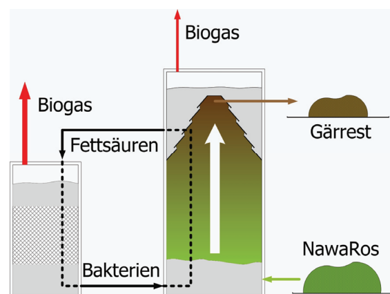
Zweistufiges Aufstromverfahren: Prozessflüssigkeit zirkuliert durch Aufstromfeststoffreaktor (re) und Festbettreaktor (li)
